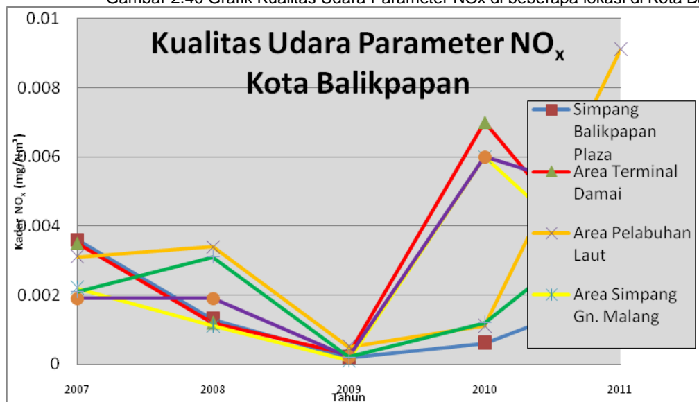
Gambar 2.40 Grafik Kualitas Udara Parameter NO x di beberapa lokasi di Kota Balikpapan
