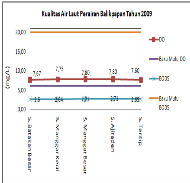
Gambar 2.51 Hasil Uji Kualitas Air Laut di Balikpapan untuk Parameter DO dan BOD5
