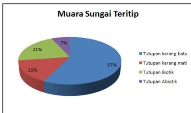
Gambar 2.58 Komposisi Terumbu karang di Muara S. Teritip
