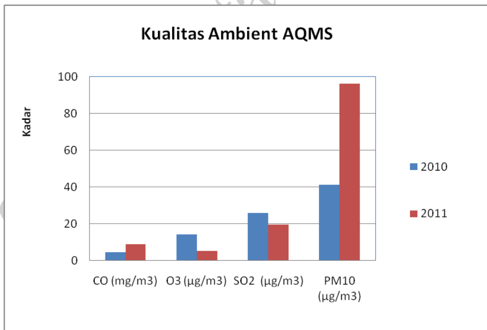
Gambar 2.44 Grafik Kualitas Udara ambient alat Pantau AQMS Tahun 2010 dan 2011
