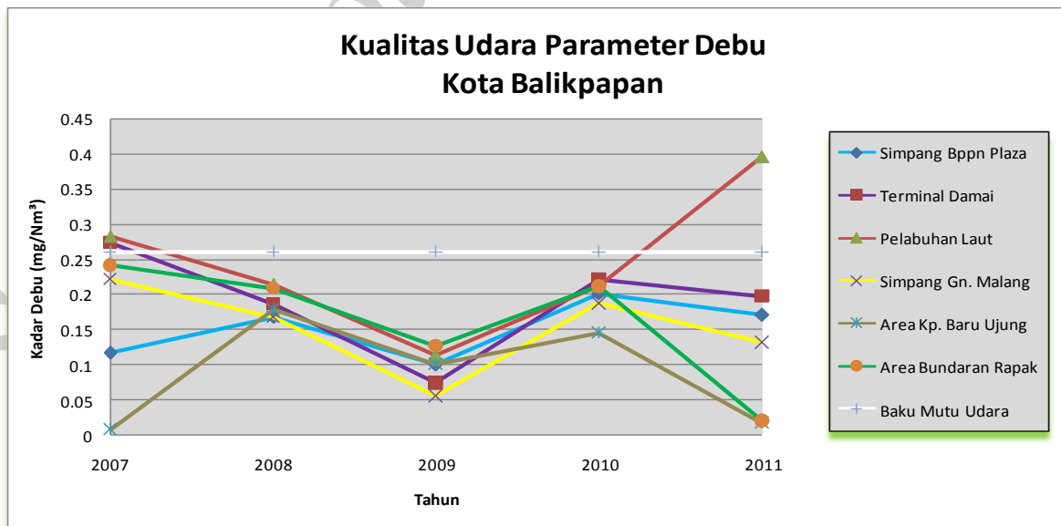
Gambar 2.36 , Grafik Kualitas Udara Parameter Debu di beberapa lokasi di Kota Balikpapan
