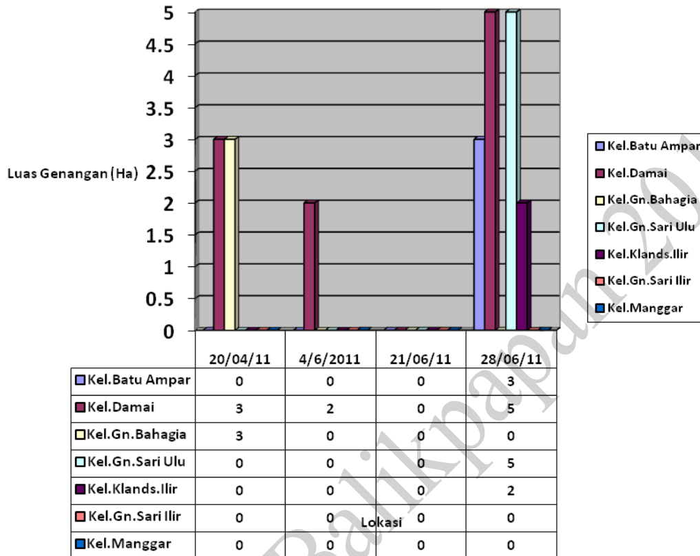
Gambar 2.61 Grafik Sebaran Luasan Banjir Januari – Juli 2011
