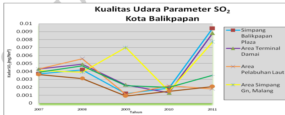
Gambar 2.37 Grafik Kualitas Udara Parameter SO 2 di beberapa lokasi di Kota Balikpapan
