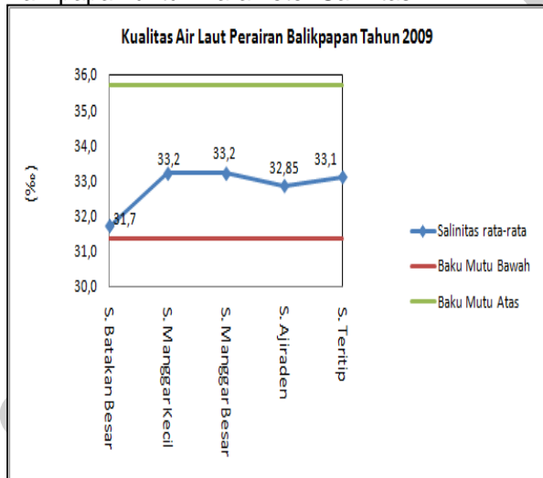
Gambar 2.52 Hasil Uji Kualitas Air Laut di Balikpapan untuk Parameter Salinitas
