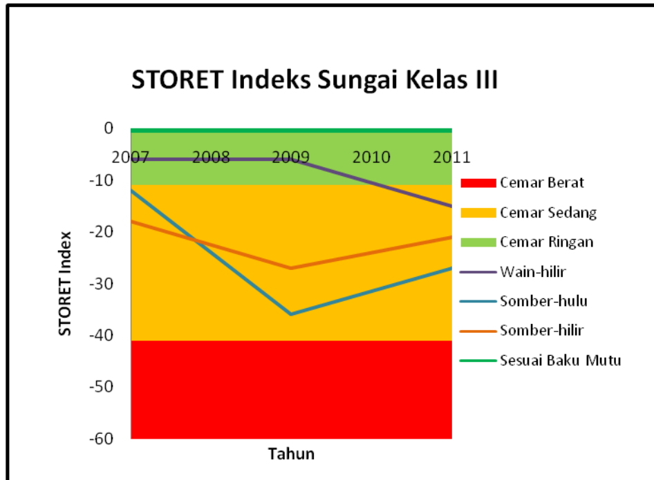
Gambar 2.35. Grafik Storet Index Baku Mutu Air Gol. III
